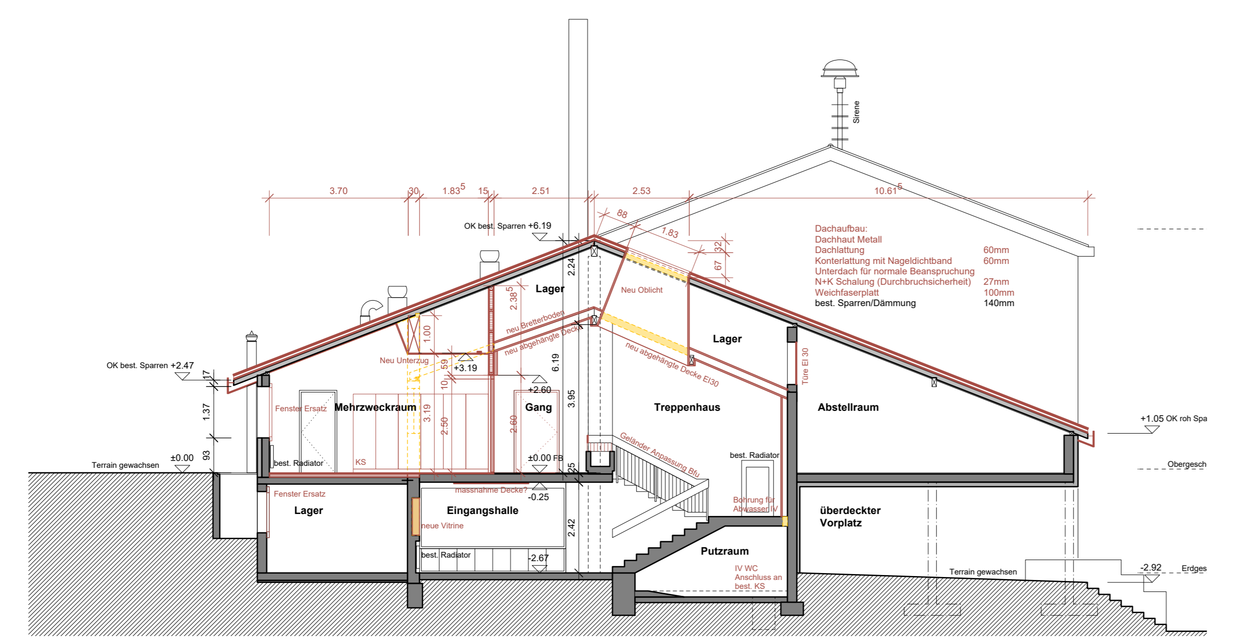
SCHNITT C
