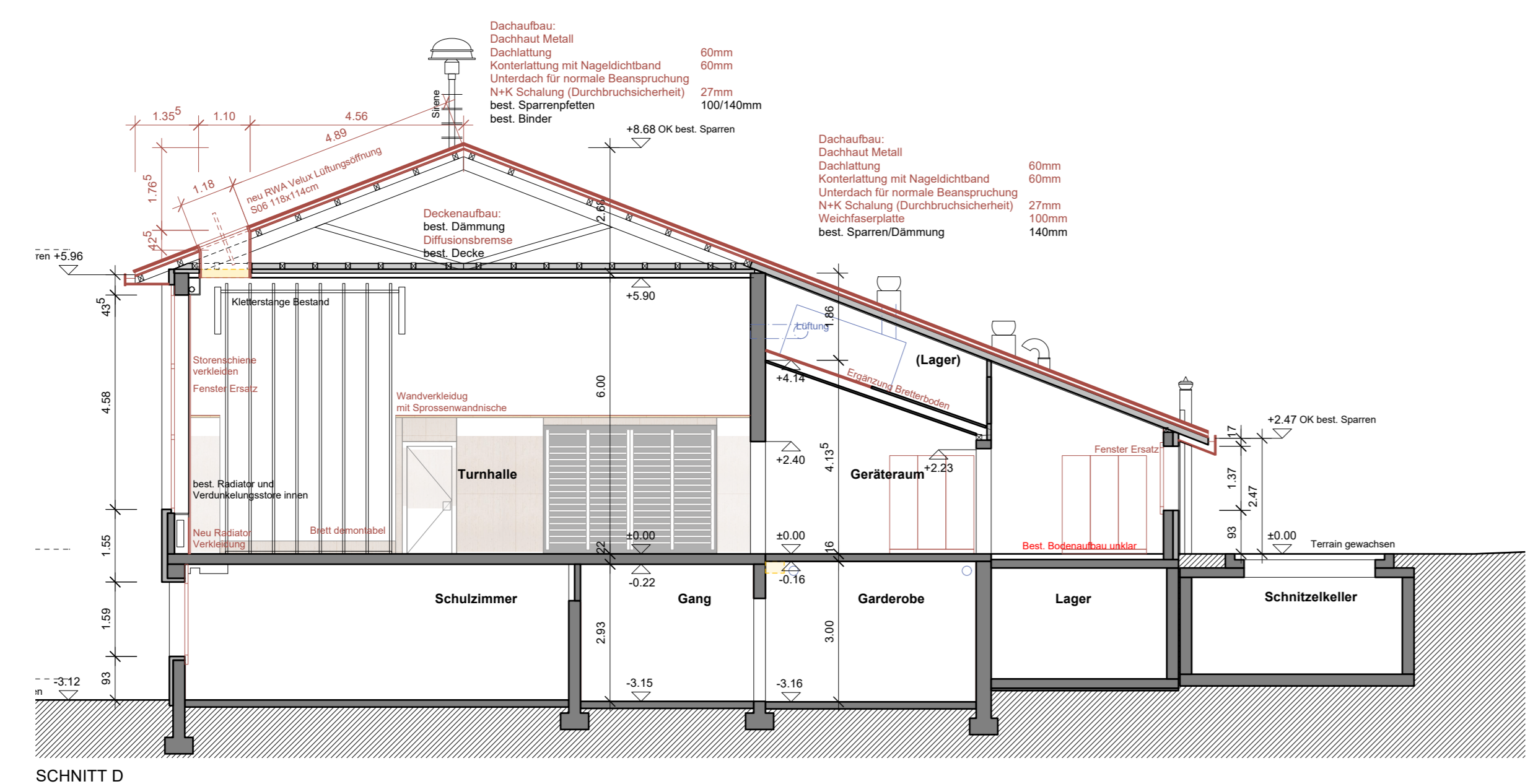
SCHNITT D
