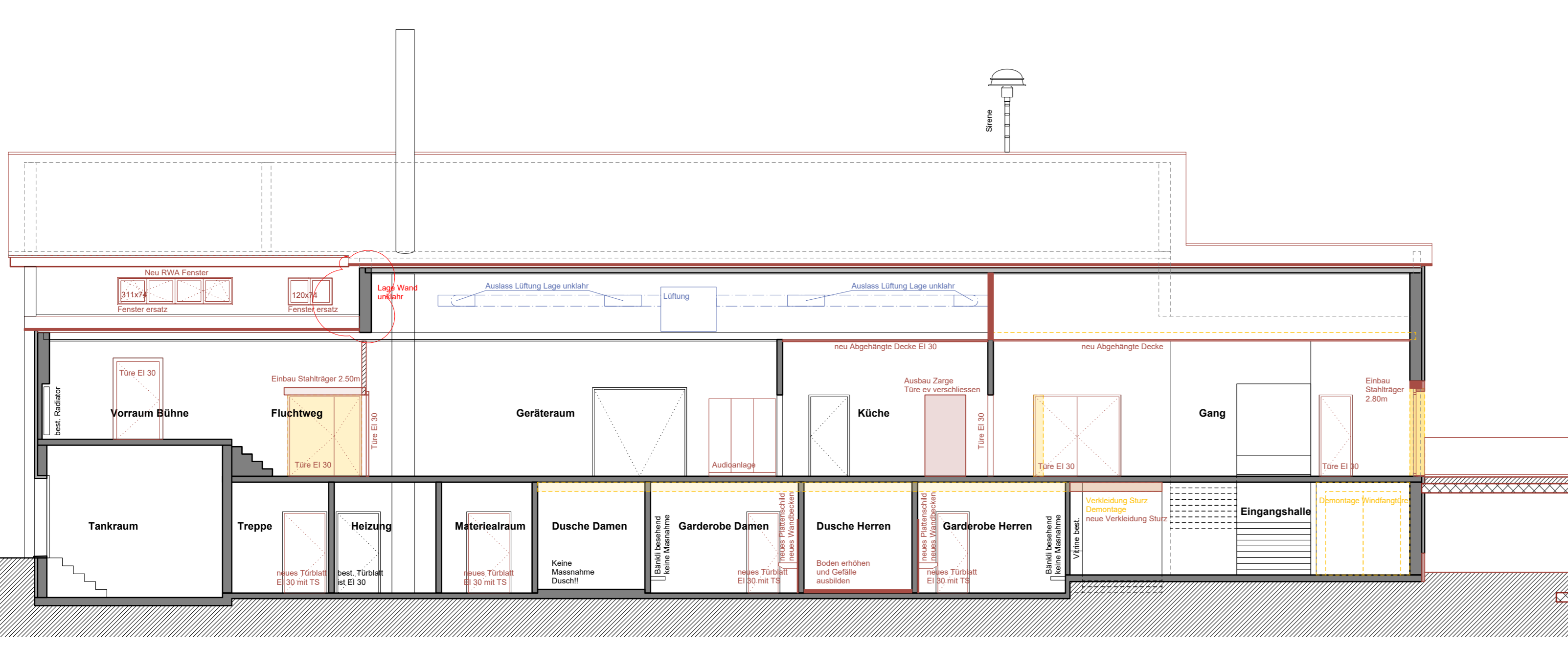
SCHNITT 1
