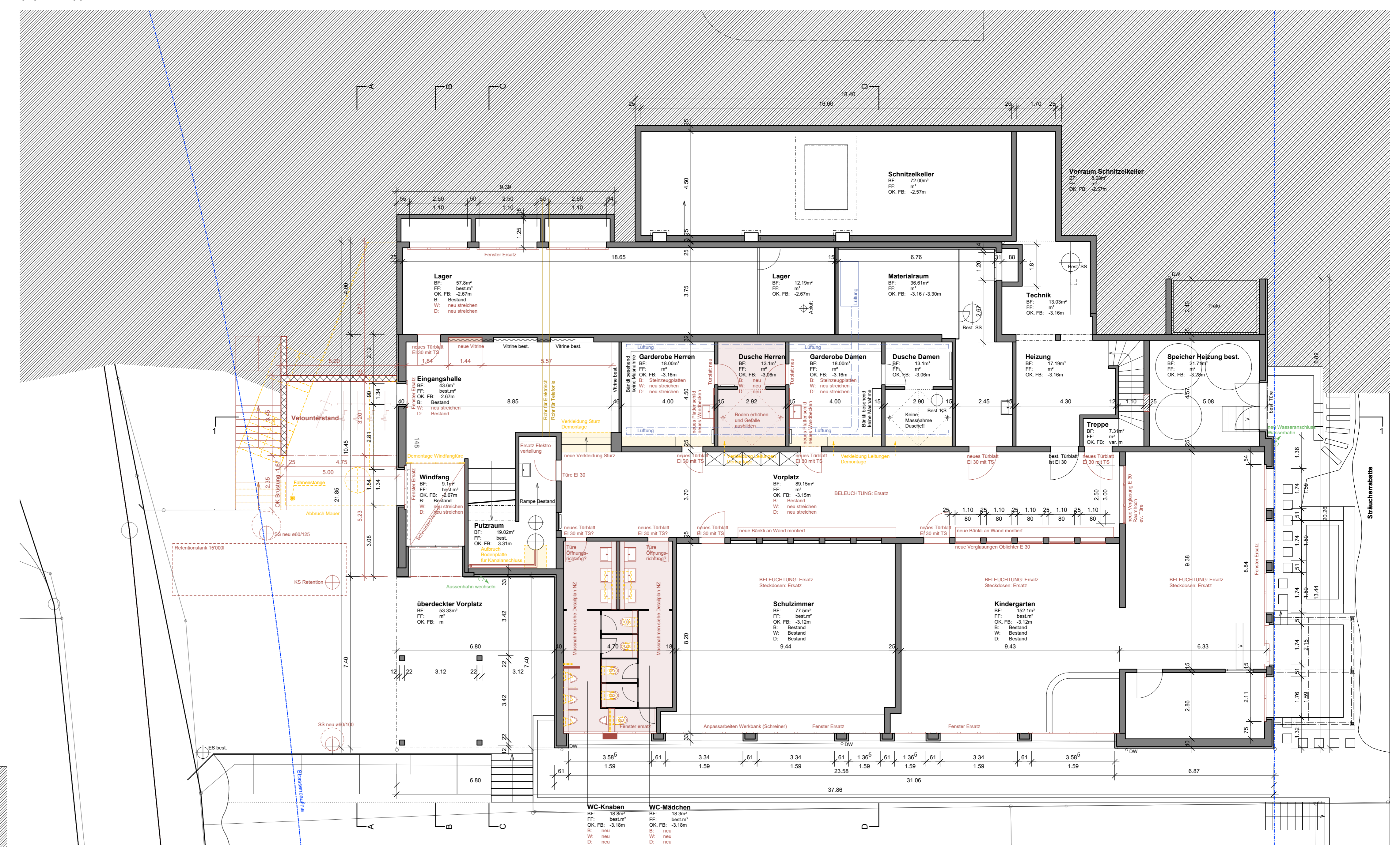
GRUNDRISS EG
